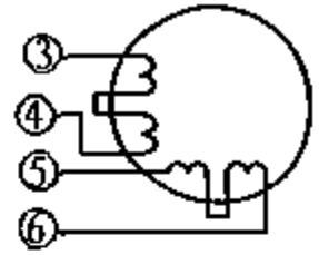
8线电机串行接法 低速力矩大
