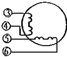
4线电机
